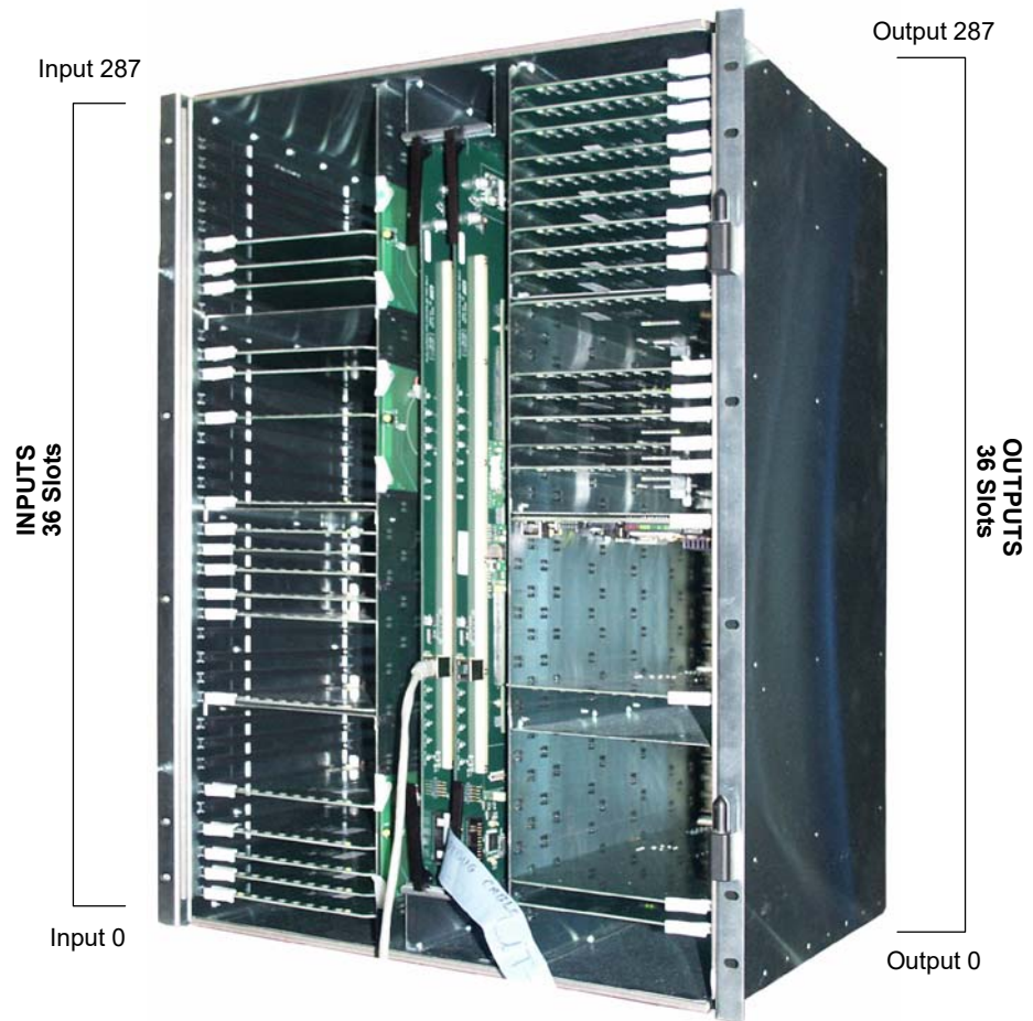
FIGURE 3-2. Module Array
